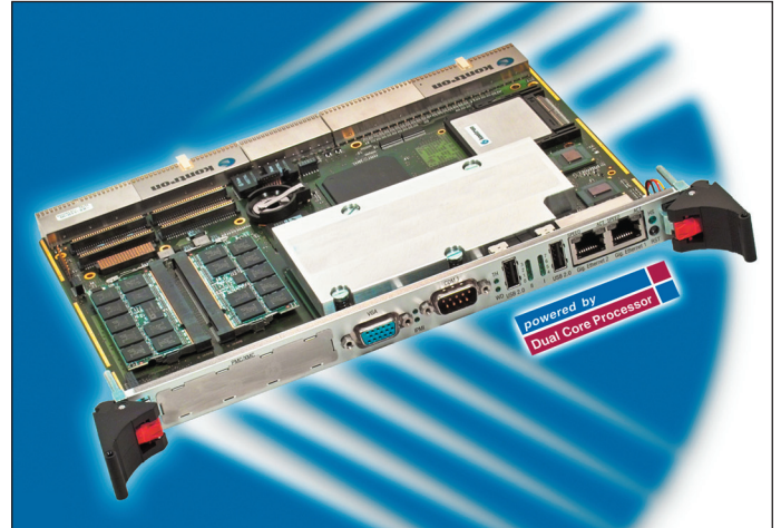
Рис. 3. Внешний вид платы Kontron CP6012
