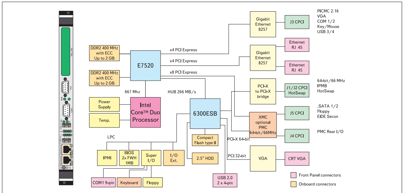
Рис. 4. Внешний вид передней панели и структурная схема Kontron CP6012. «Наплатные» гнезда и соединители выделены коричневым цветом, разъемы и порты, выведенные на переднюю панель, — лиловым
