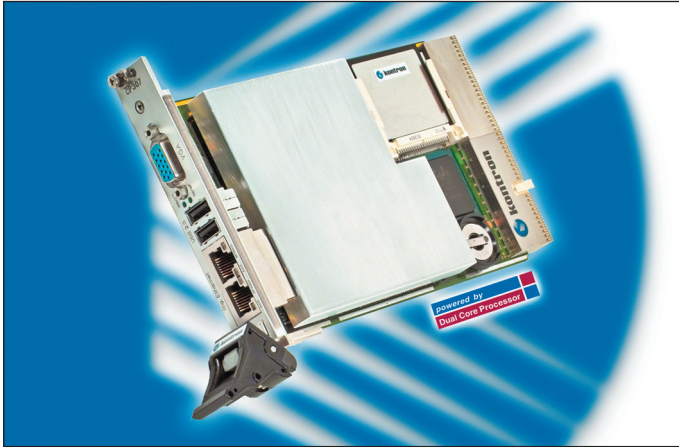
Рис. 1. Модуль Kontron CP307, реализованный в конструктиве 3U CompactPCI на базе двудядерного процессора Intel Core Duo
