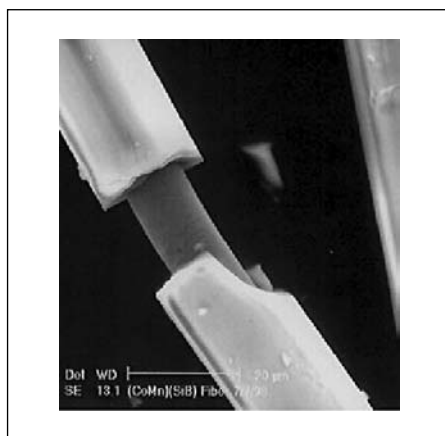
Рис. 2. Электронная микрофотография строения аморфного ферромагнитного микропровода в стеклянной изоляции (длина масштабного штриха на снимке — 20 мкм)
