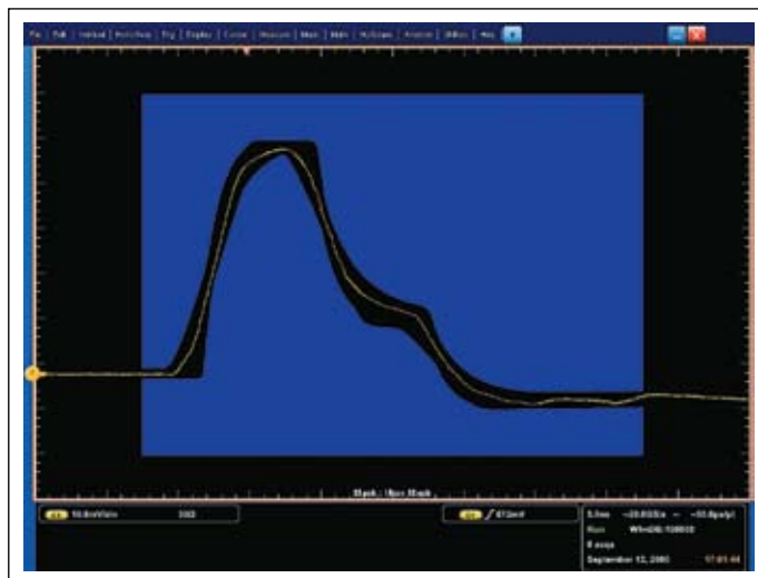
Рис. 4. Тестирование по маске сигналов стандарта Ethernet
