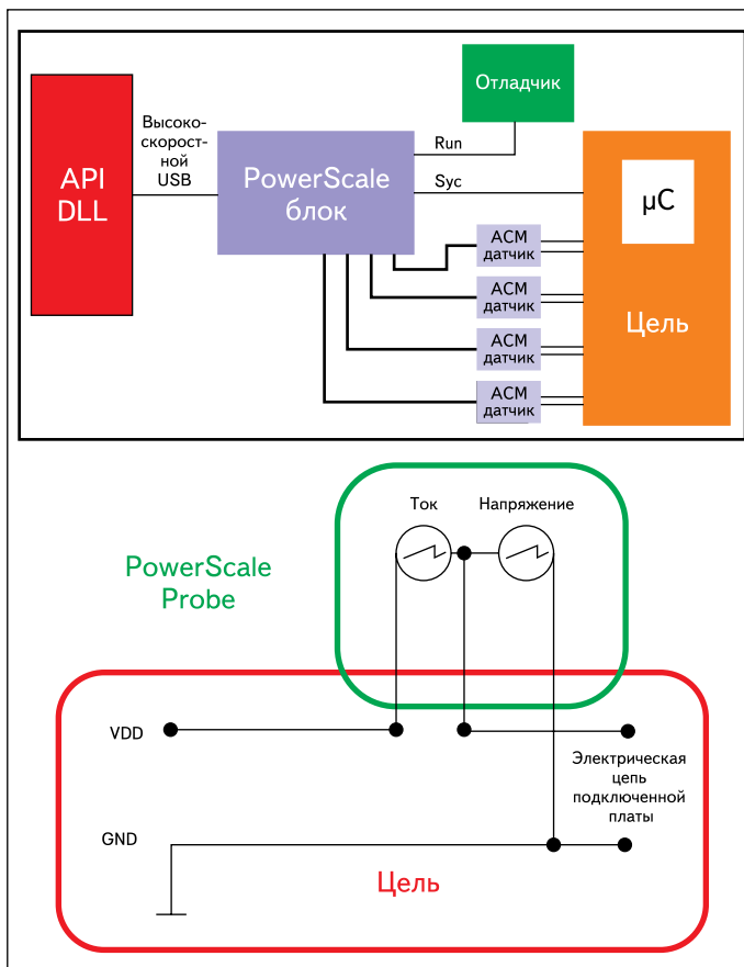
Рис. 2. Подключение PowerScale и датчиков
