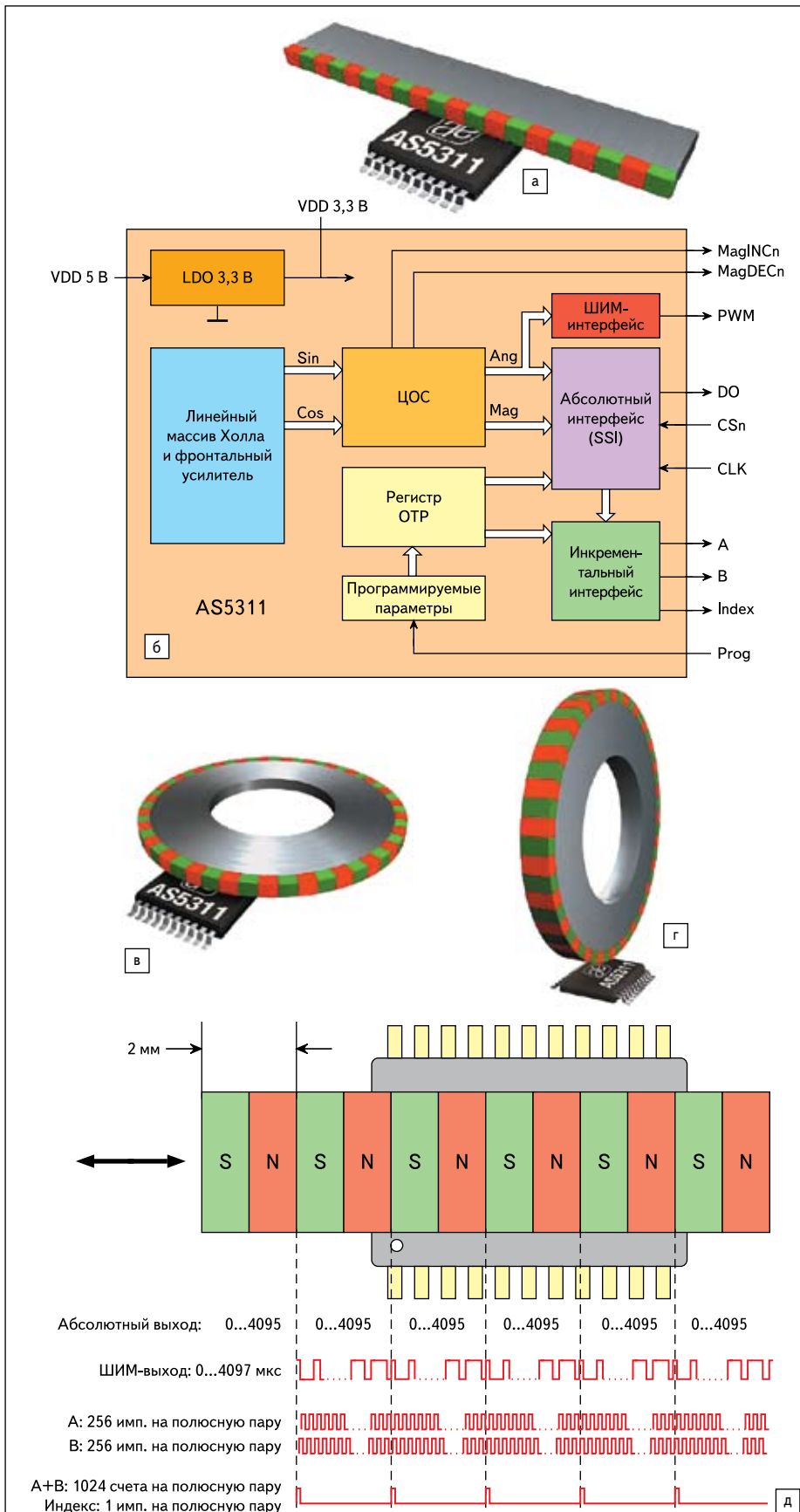
Рис. 5. Эncoder AS5311 Austriamicrosystems — новая ИС Холла для линейного и углового Off-Axis детектирования движения многополюсного магнита: а) рабочий режим, для которого разрабатывалась ИС; б) функциональная диаграмма датчика; в, г) альтернативные угловые рабочие режимы с многополюсным кольцевым магнитом; д) диаграммы выходных сигналов при перемещении механической части ротора
