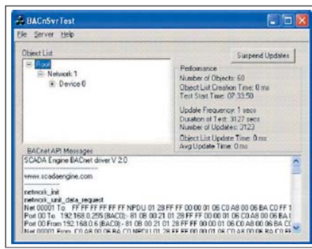
Рис. 4. Пример работы симулятора ВАСnet
