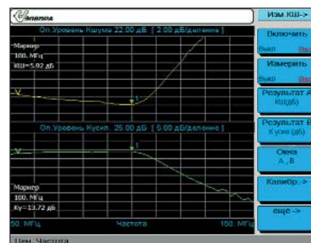
Рис. 14. Интерфейс программного обеспечения для измерения КШ в «СК4-БЕЛАН 32»
