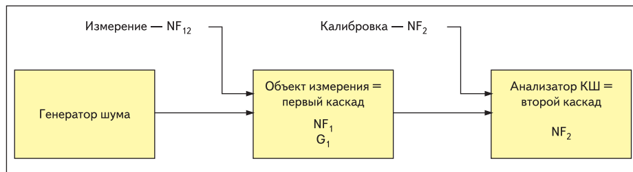
Рис. 10. Двухкаскадная система
