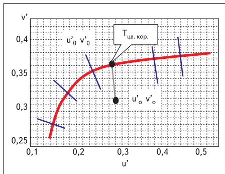
Рис. 3. Линия АЧТ в системе цветовых координат u', v'
