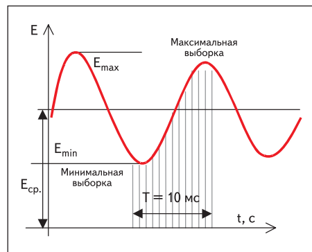
Рис. 4. Временная характеристика пульсирующей освещенности
