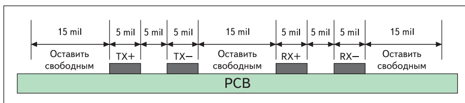
Рис. 8. Примеры расположения трасс сигналов TX и RX
