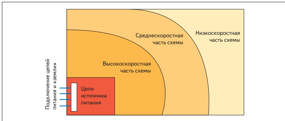
Рис. 9. Расположение компонентов на печатной плате в зависимости от скорости работы цепей
