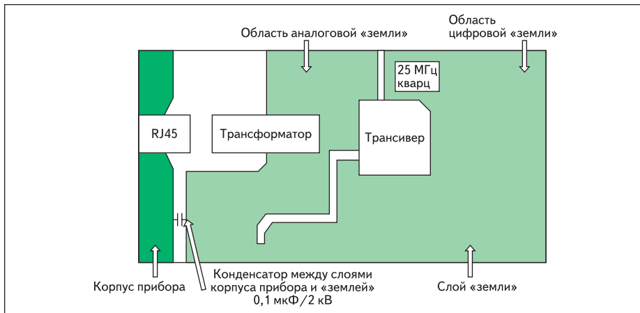
Рис. 3. Расположение областей цифровой и аналоговой «земли»
