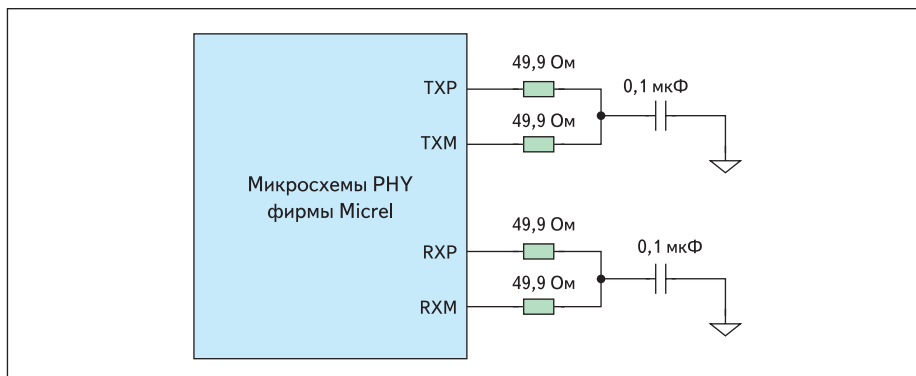
Рис. 7. Согласование цепей TX и RX
