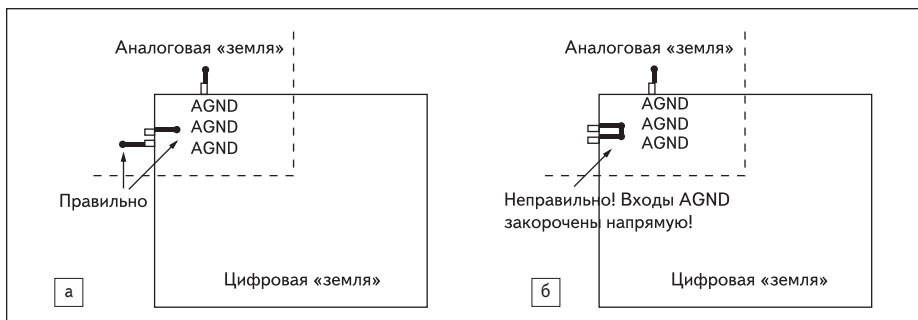
Рис. 4. Подключение выводов микросхемы к аналоговой «земле»
