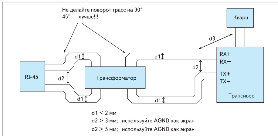
Рис. 6. Расположение компонентов и трасс на плате
