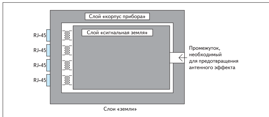
Рис. 2. Расположение слоя «земли» и «корпуса»
