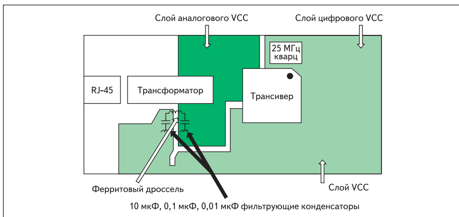
Рис. 5. Расположение областей цифрового и аналогового питания
