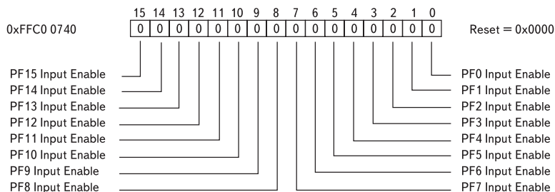
Рис. 7. Биты регистра разрешения входов флагов FIO_INEN
