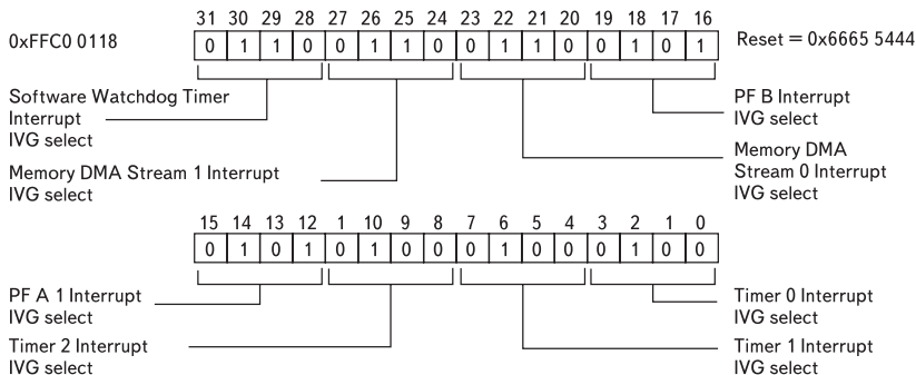
Рис. 8. Биты регистра назначенных прерываний SIC_IAR2
