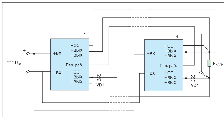
Рис. 5. Схема параллельного включения модулей МДМ-ВТ
