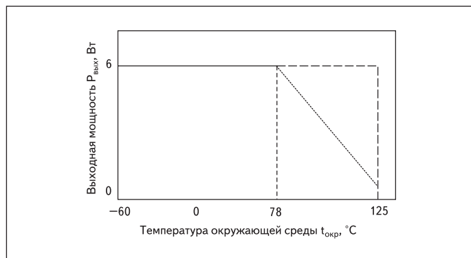
Рис. 4. График снижения мощности
