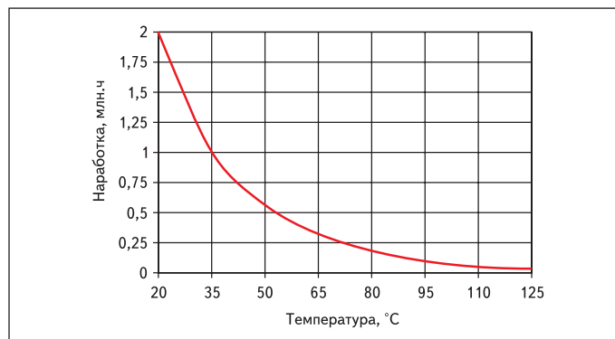
Рис. 6. График зависимости наработки на отказ от температуры
