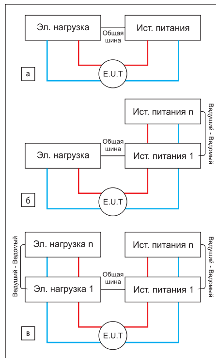
Рис. 3. Пример реализуемых систем тестирования и испытания: а) конфигурация из 1 нагрузки и 1 источника; б) конфигурация из 1 нагрузки и N+1 источников; в) конфигурация из N+1 нагрузок и N+1 источников
