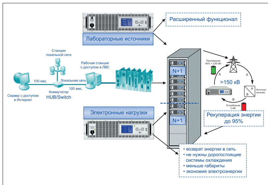
Рис. 4. Пример реализации системы тестирования (N+1) с рекуперацией энергии и компьютерным управлением
