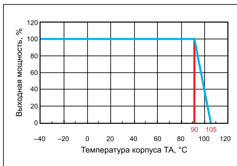
Рис. 11. Зависимость выходной мощности модулей серии ВА от температуры корпуса
