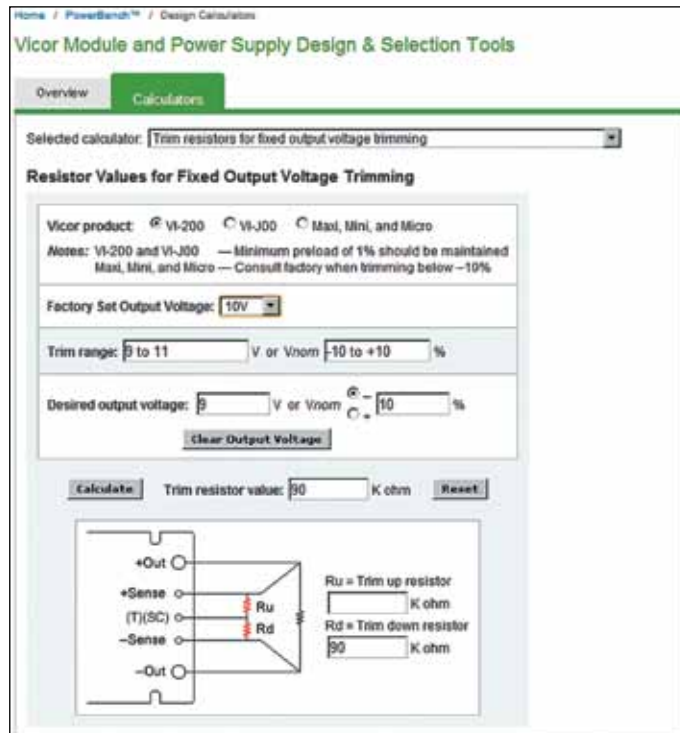
Рис. 6. Фрагмент рабочего экрана калькулятора для расчета сопротивлений резисторов, задающих фиксированное выходное напряжение
