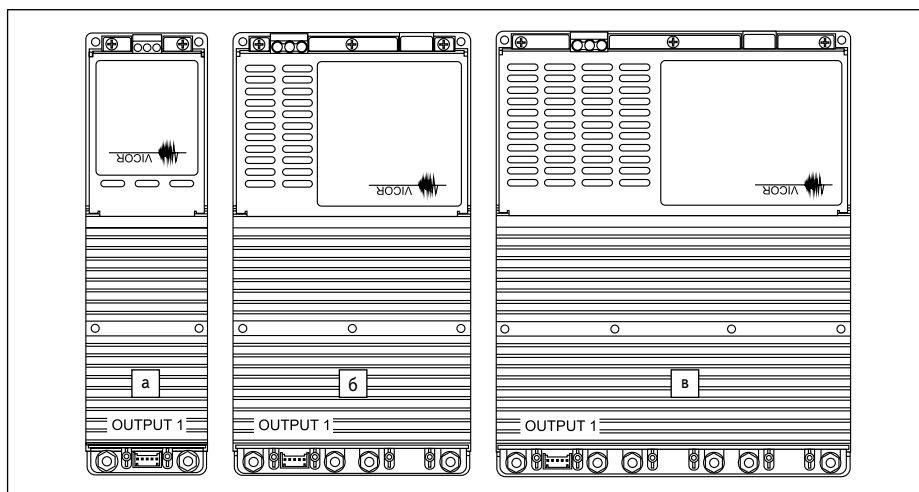
Рис. 2. Внешний вид корпуса (вид сверху): а) 1-UP; б) 2-UP; в) 3-UP
