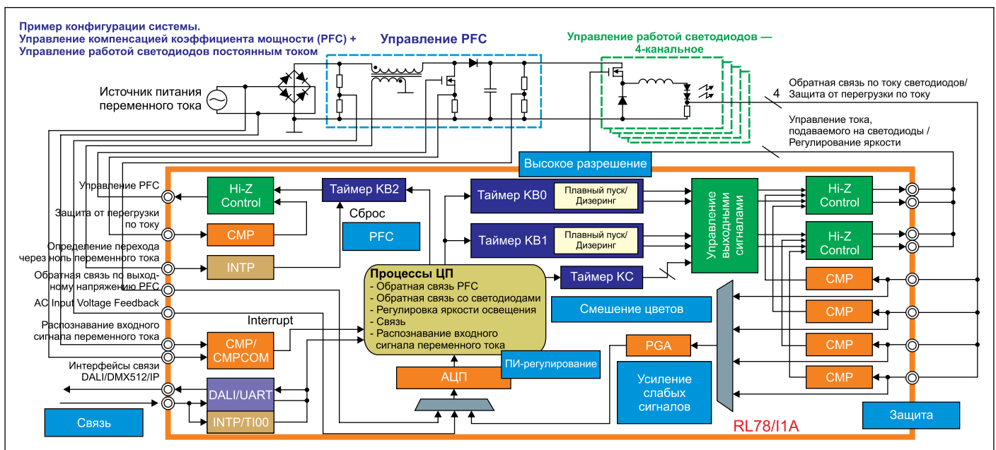
Рис. 2. Блок-схема микроконтроллера RL78/11A с типичным примером его применения в качестве светодиодного драйвера
