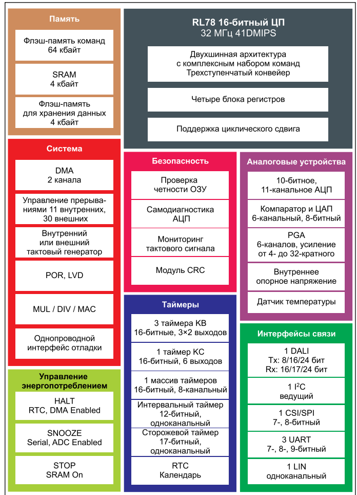
Рис. 1. Блок-схема микроконтроллера RL78/11A
