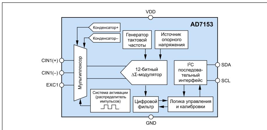
Рис. 5. Функциональная схема микросхемы AD7153
