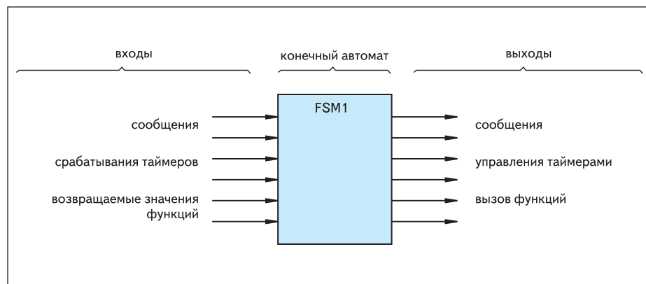
Рис. 1. Конечный автомат с входами и выходами
