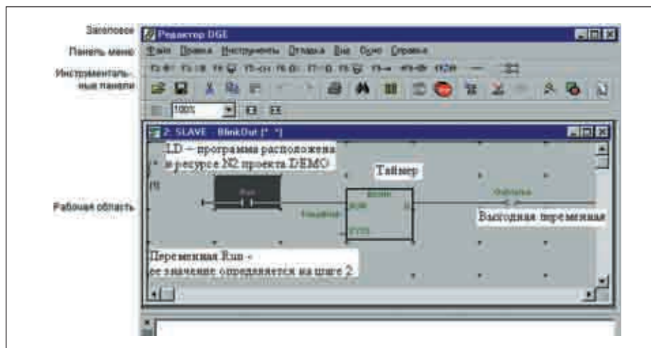
Рис. 6. Вид редактора DGE и программа BlinkOut ресурса Slave
