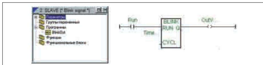
Рис. 7. Ресурс 2 и программа LD
