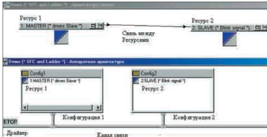
Рис. 1. Структура проекта Demo
