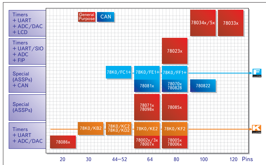
Рис. 3. Микроконтроллеры серии 78K0
